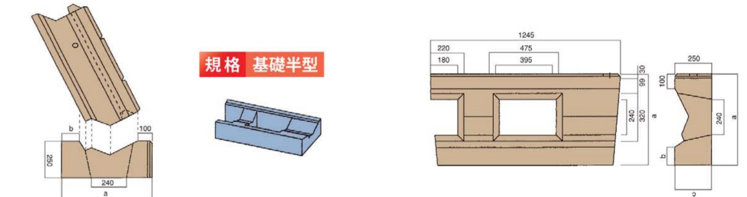
■寸法表(5分勾配)
